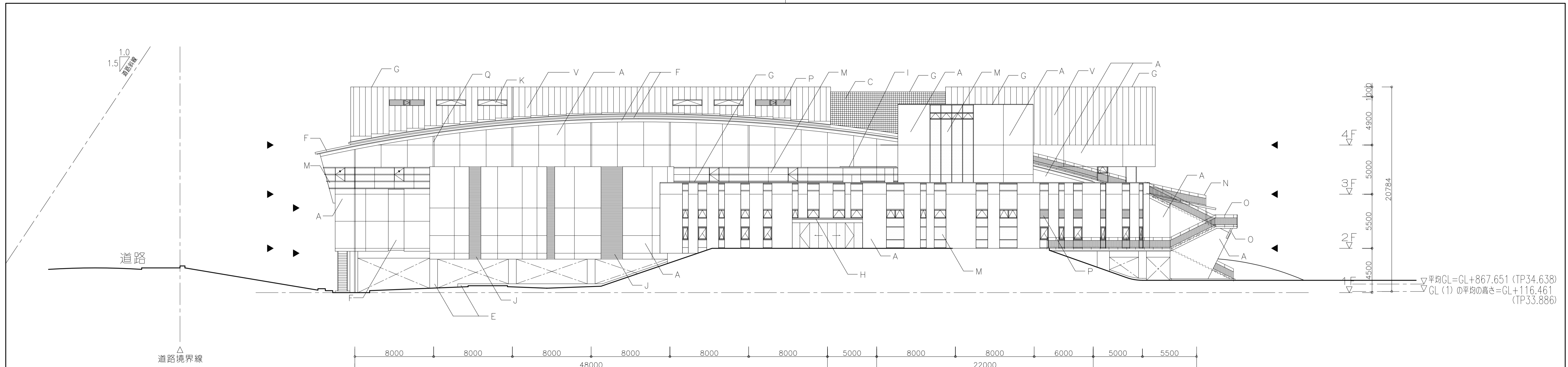
西側立面図
