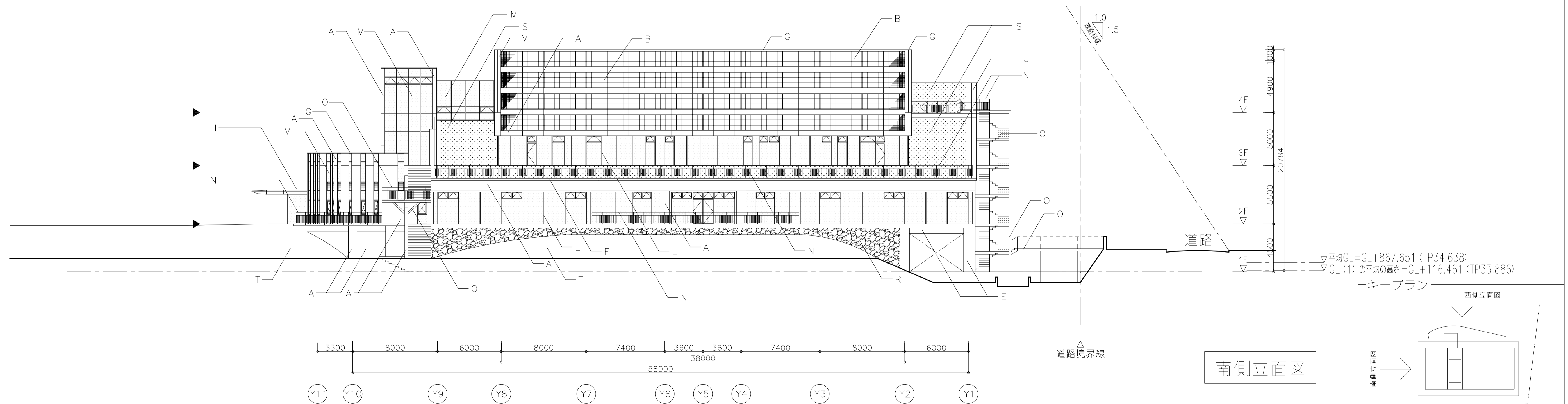
南側立面図 (X2部分)
