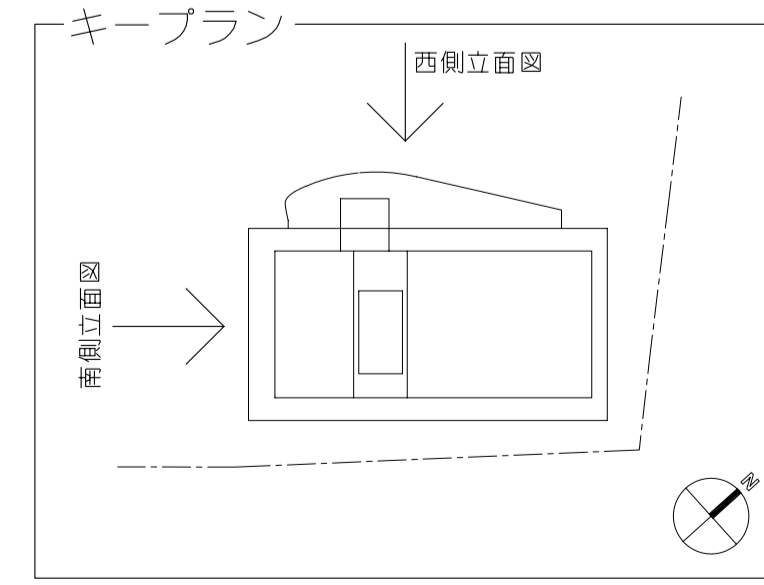
南側立面図
