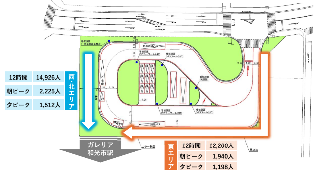
※R6.3.28都市計画決定時点の駅前広場計画図
