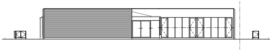
南立面图 S = 1 / 200
