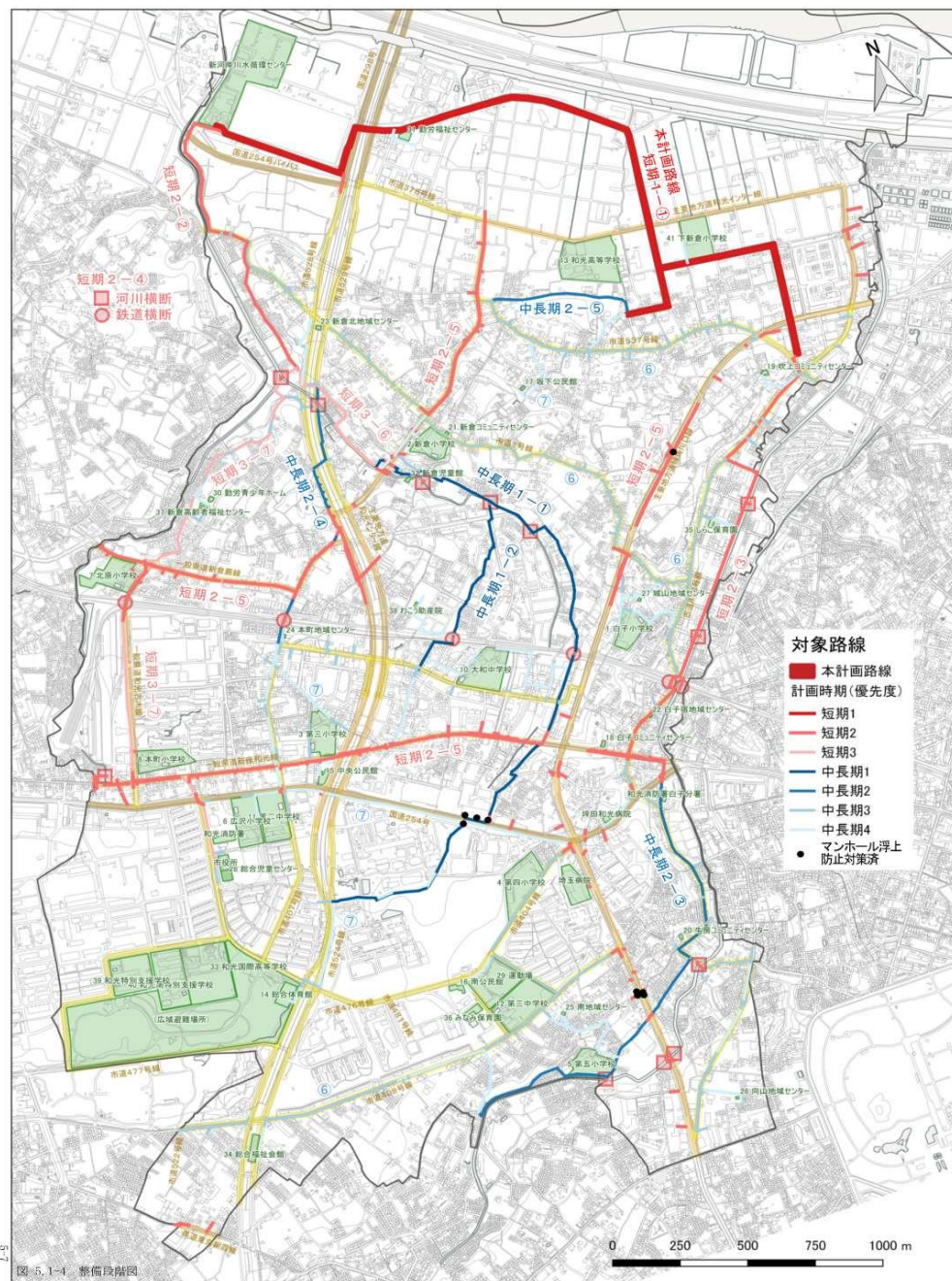
図5.1-4 整備段階図
